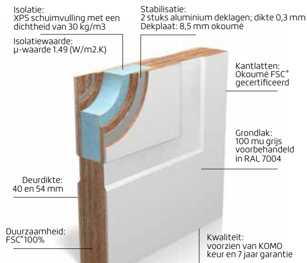
Skantrae Nova Panel
