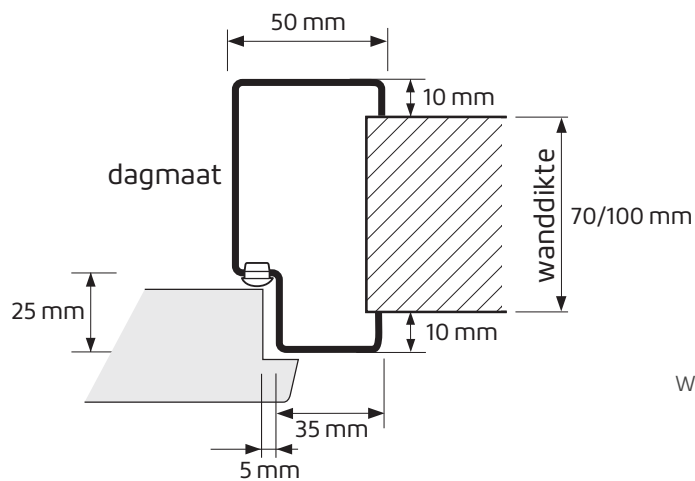
Profiel opdekuitvoering
